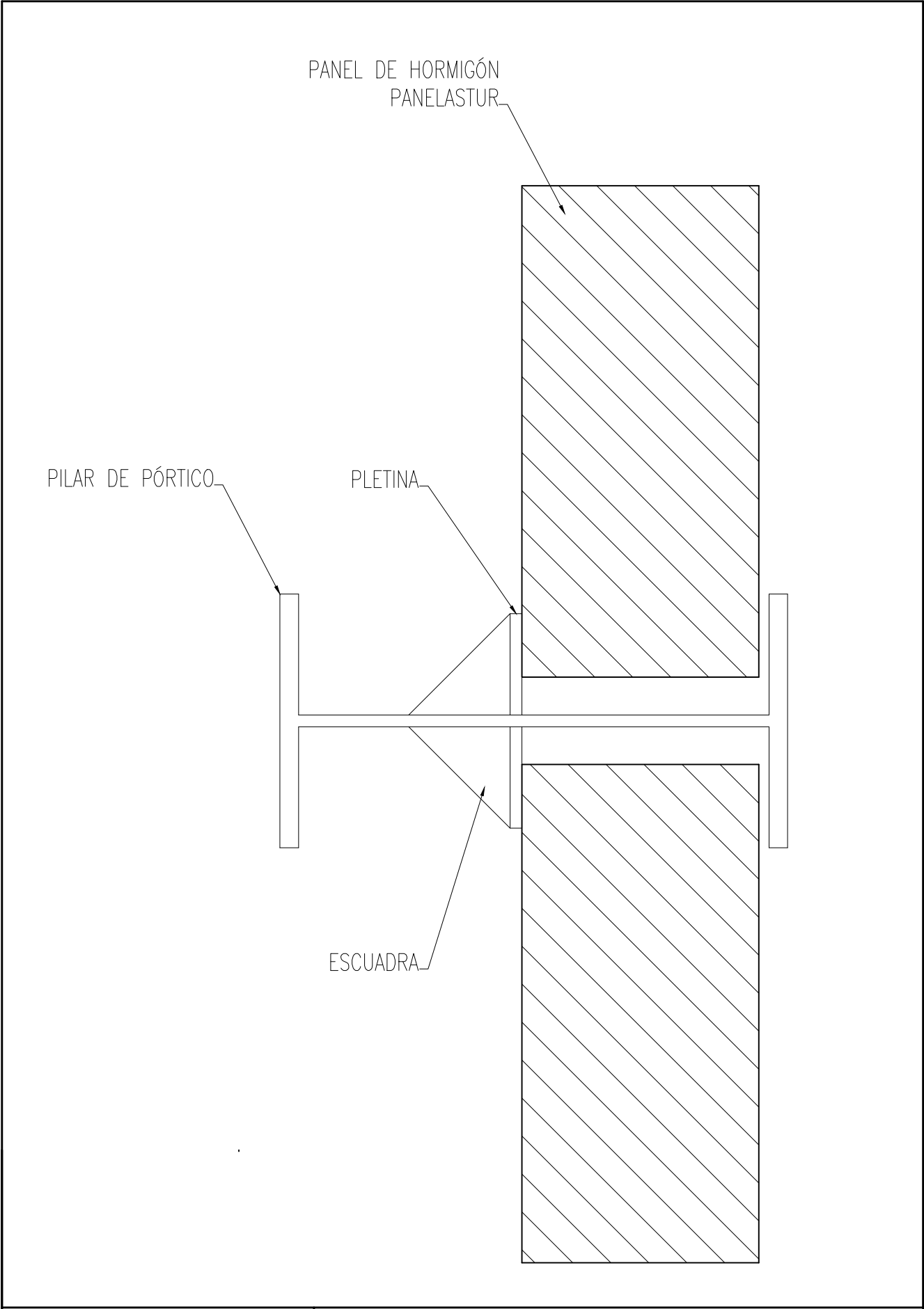
DETALLE SUJECCIÓN PANELES ENTRE PILARES
